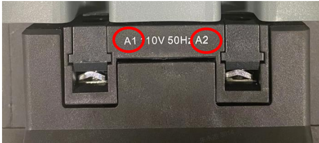
NXCC-150~170 切换电容器接触器（俯视）：
