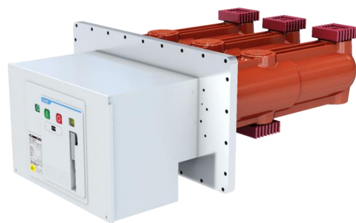
NV77-40.5/T4000-40 真空断路器 (配充气柜)
